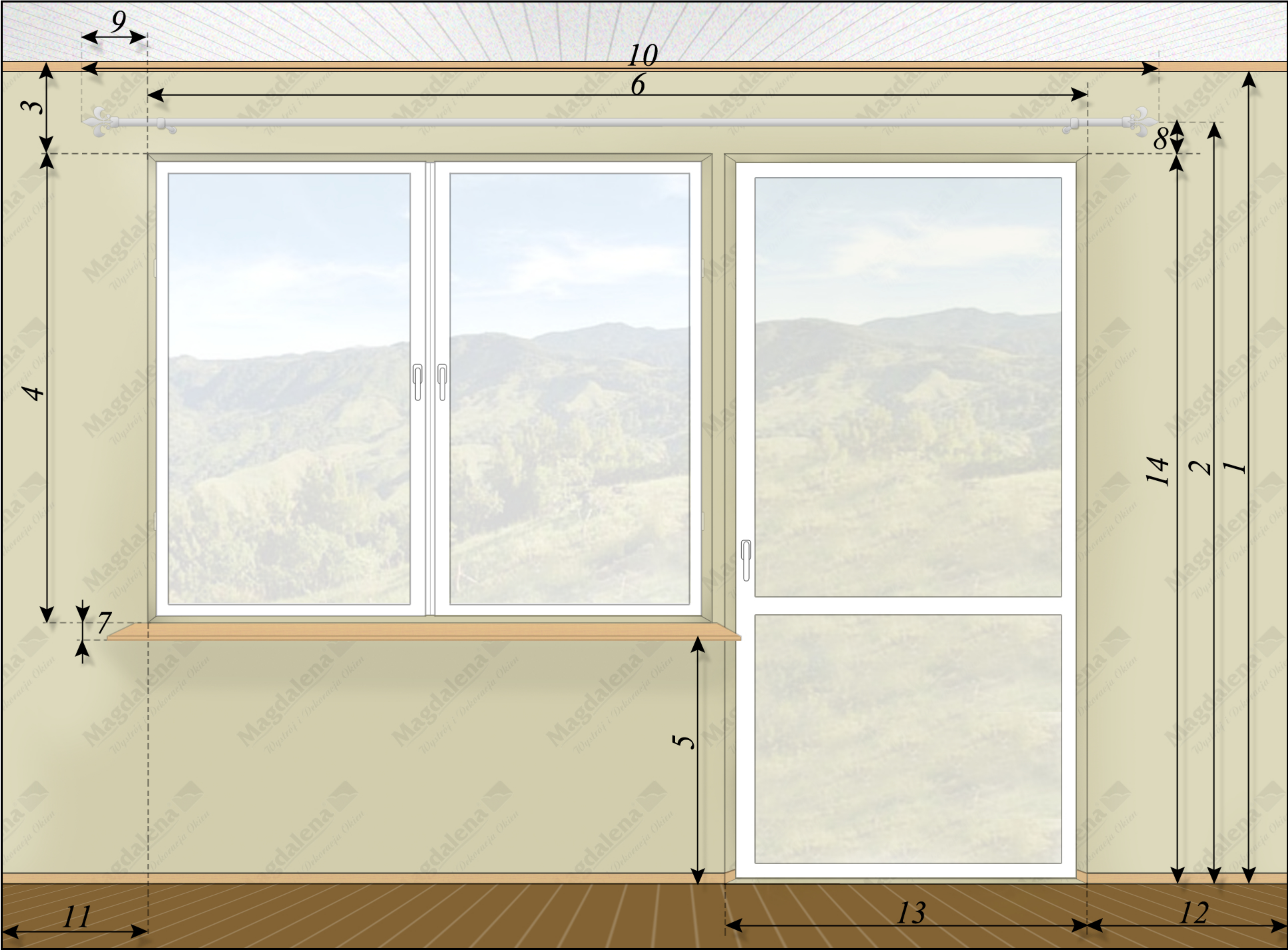
Rys. Schemat pomiaru okna i drzwi balkonowych
